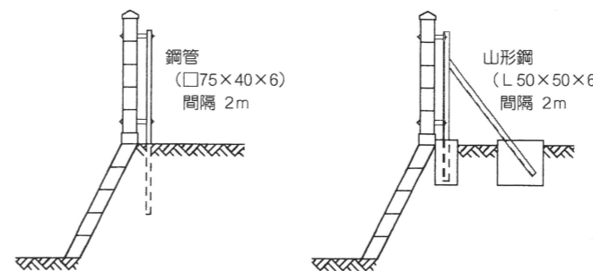
① 鋼柱(鋼管)式 ② 鋼柱(山形鋼)式
