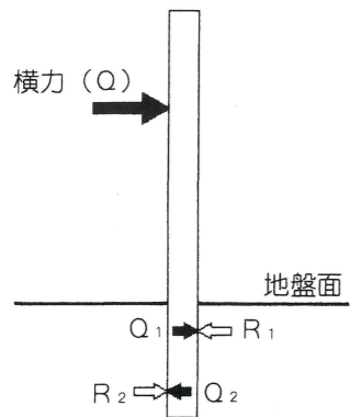
基礎における力の釣合モデル
