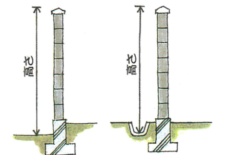
ブロック塀の高さの測り方
