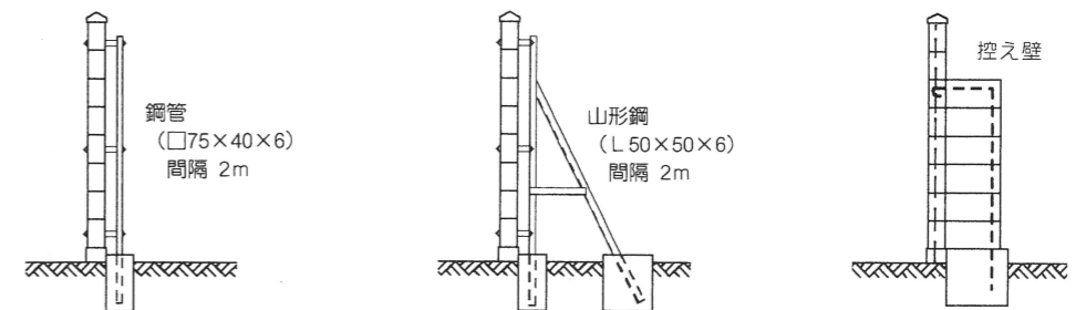
① 鋼柱(鋼管)式 ② 鋼柱(山形鋼)式 ③ 控え壁式
